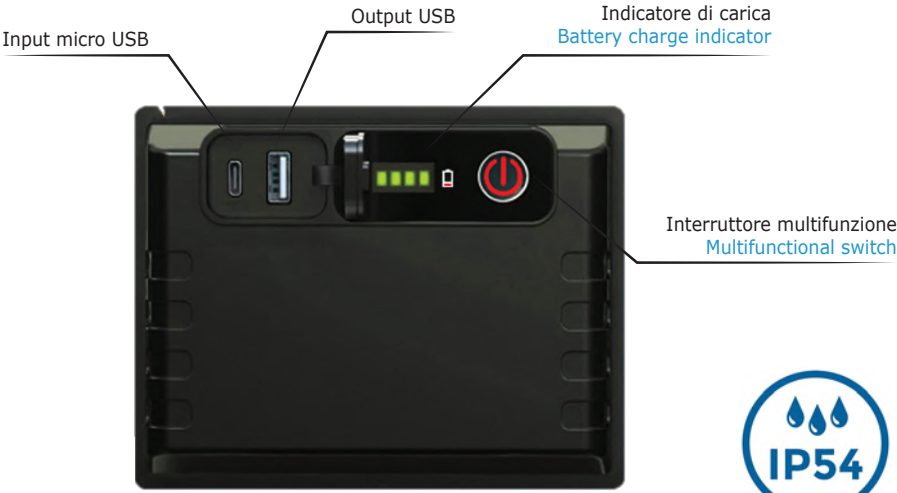
VB-CA-USB Alimentatore USB USB power supplier USB 230V, 5 VDC, 1A, 5W
